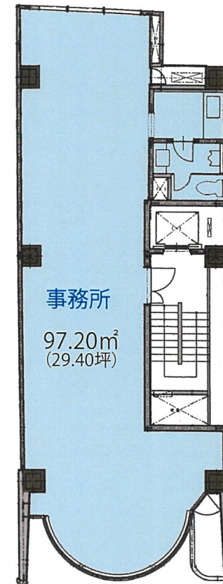
◆ 5階平面図
